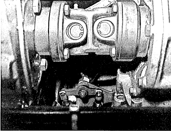
Bild 30 Gelenkwelle
