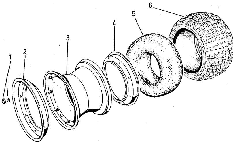
Bild 37 Lypsoïd-Reifen
