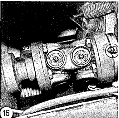
Bild 131 Kreuzgelenke für Antriebsachse
