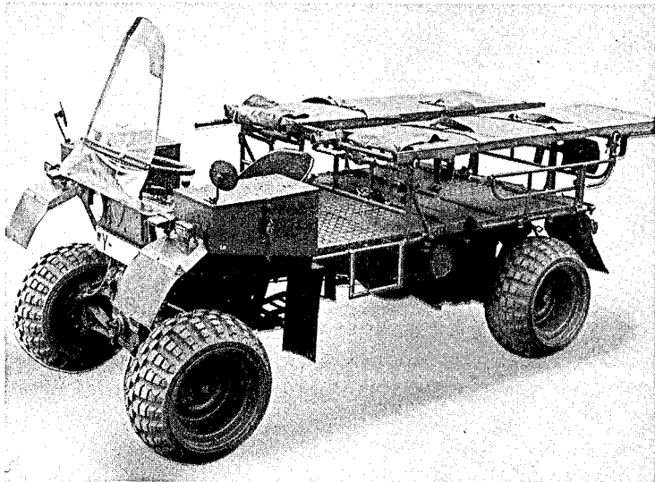
Bild 51 Fahrzeug mit aufgebauten Krankentragen
