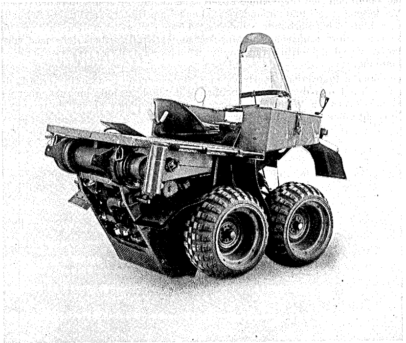
Bild 44 Fahrzeug zusammengeklappt
