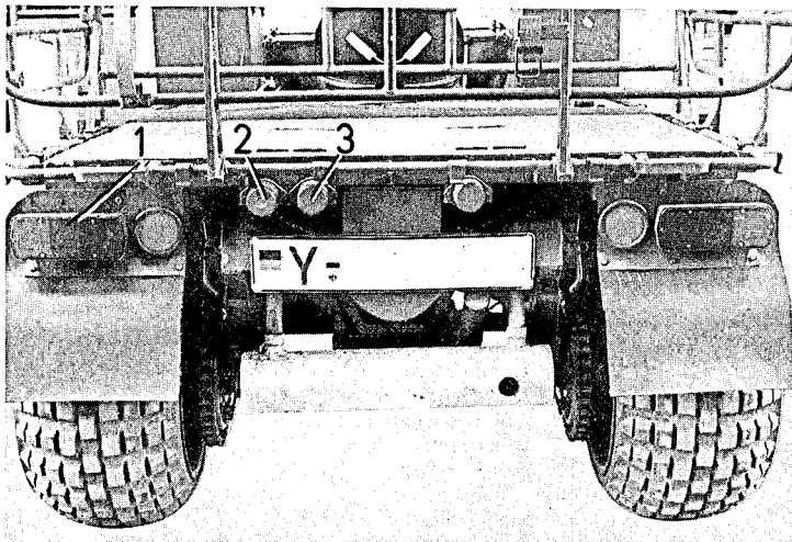
Bild 26 Beleuchtungsanlage hinten
