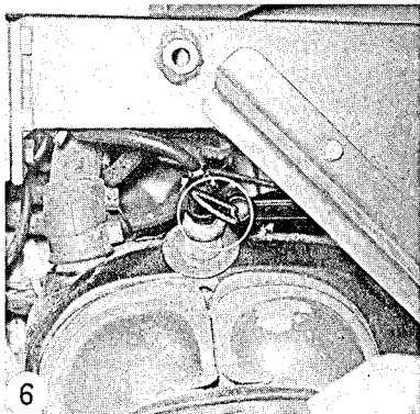
Bild 120 Motorölmeßstab
