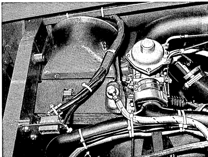
Bild 12 Ölkühler mit elektrischem Gebläse
