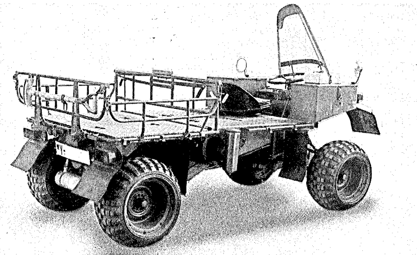
Bild 2 Ansicht hinten rechts
