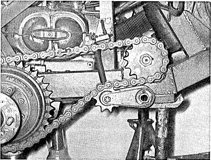
Bild 38 Antriebskette (das Hinterrad ist abgenommen)
