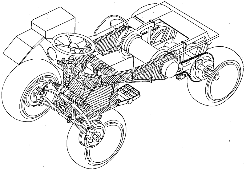
Bild 42 Fahrgestell, Vorderwagen
