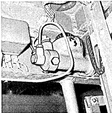
Bild 33 Hauptbremszylinder mit Ausgleichbehälter
