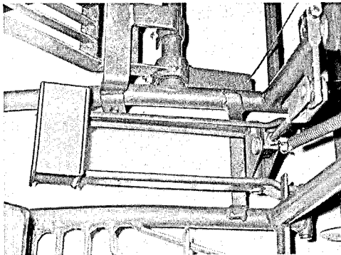
Bild 75 Bremspedal
