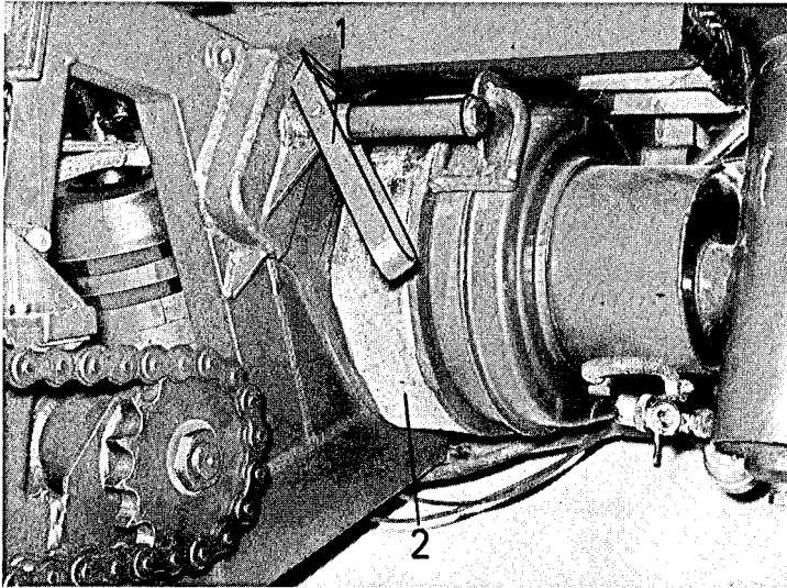
Bild 45 Ringförmiges Federelement und Schnellverschuß
