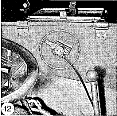
Bild 127 Seilzug für Starterklappe (am Hebel)
