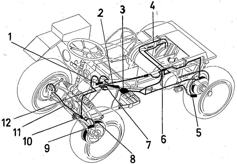
Bild 36 Schema der hydraulischen und mechanischen Bremsanlage
