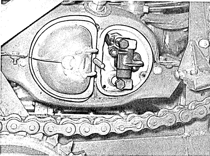
Bild 11 Zylinderköpfe (1 Ventildeckel abgenommen)
