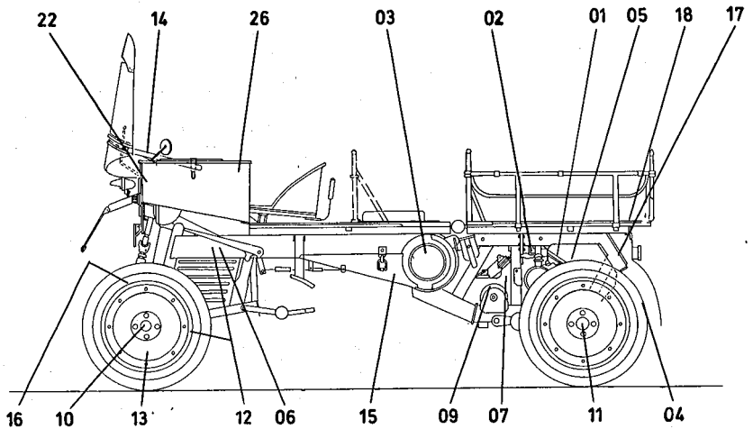
Bild 5 Baugruppenübersicht
