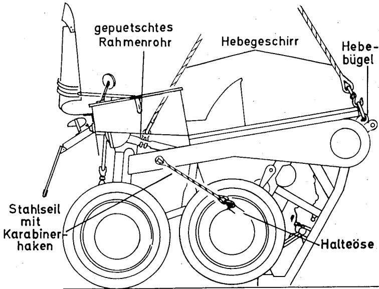
Bild 109 Verlastung Fahrzeug zusammengeklappt
