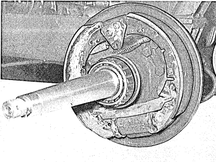
Bild 35 Radbremse (die Bremstrommel ist abgenommen)
