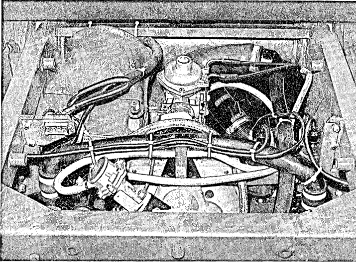
Bild 9 Motoransicht hinten (Ladebrücke abgenommen)
