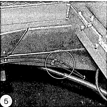
Bild 119 Seilzüge für Gasbetätigung und Starterklappe
