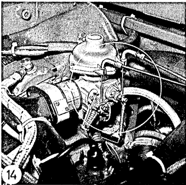
Bild 129 Seilzüge für Gasbetätigung und Luftklappe (am Vergaser)
