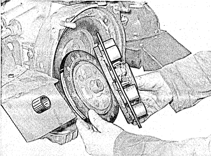
Bild 13 Einscheiben-Trockenkupplung
