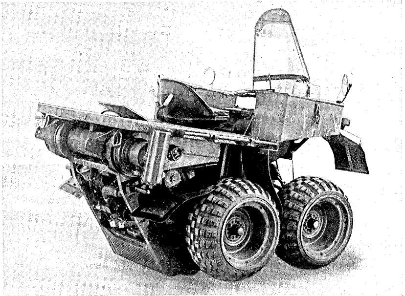
Bild 4 Ansicht hinten rechts, zusammengeklappt
