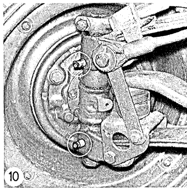
Bild 124 Achsschenkel
