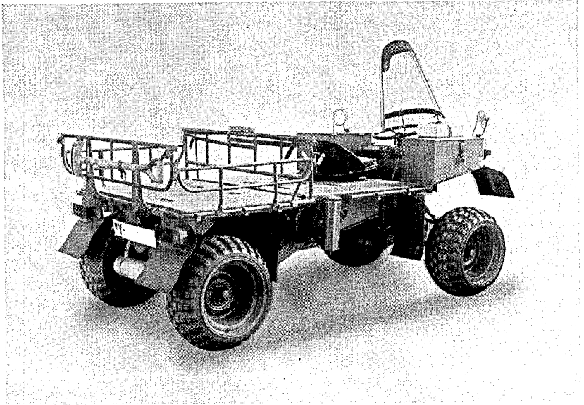
Bild 50 Hinterwagen mit Ladebrücke
