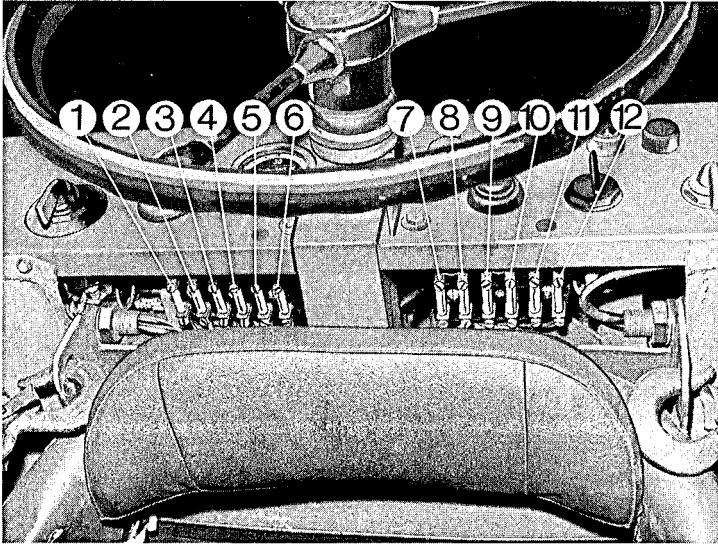
Bild 23 Schmelzeinsatzanordnung
