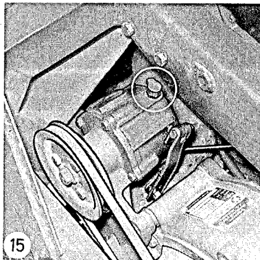
Bild 130 Drehzahlbegrenzer
