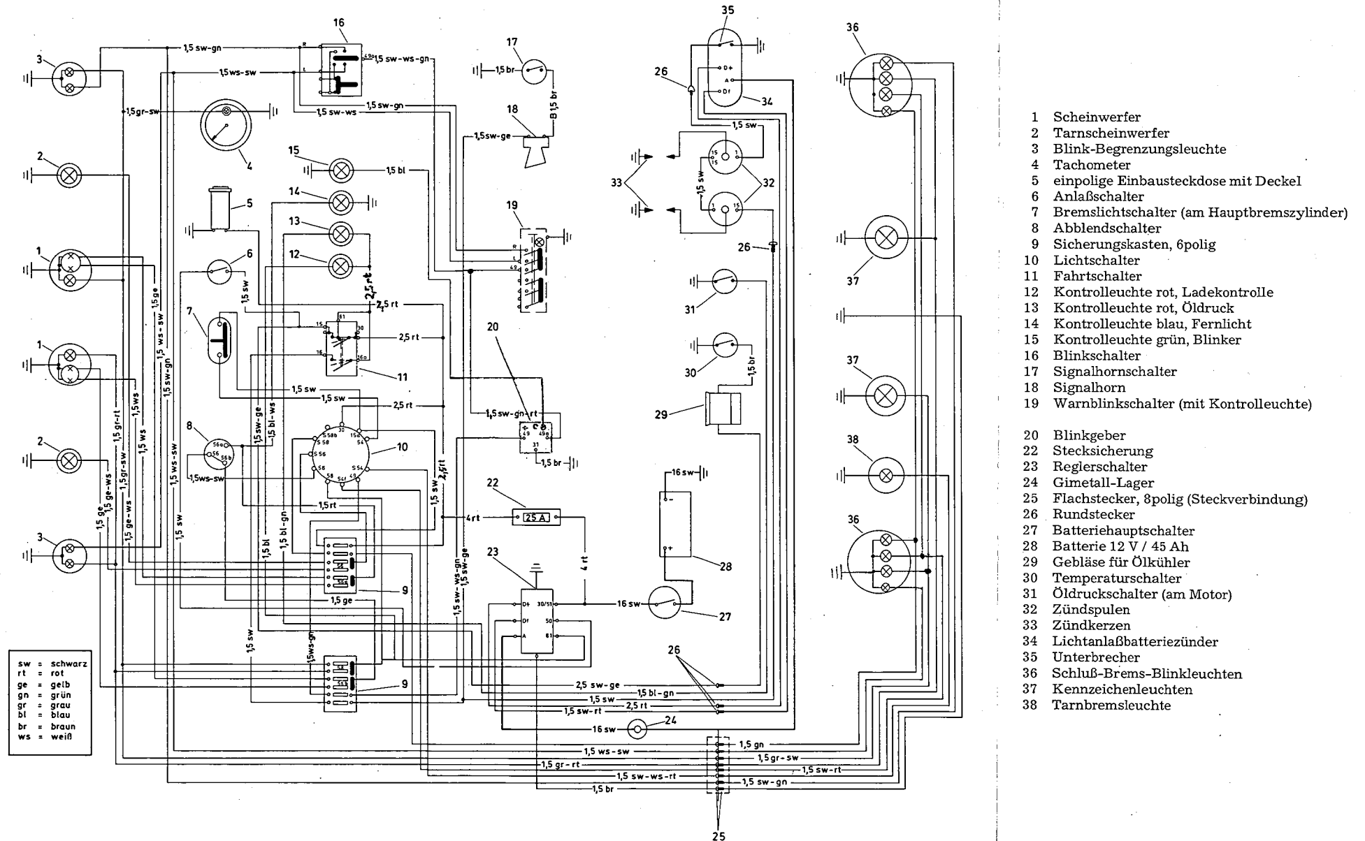
Bild 28 Wirksaltplan der elektrischen Anlage
