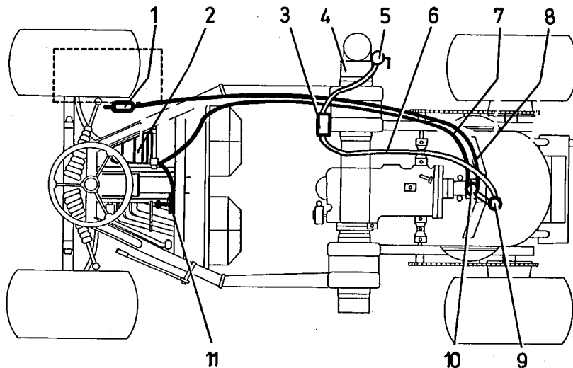
Bild 15 Schema der Kraftstoffanlage
