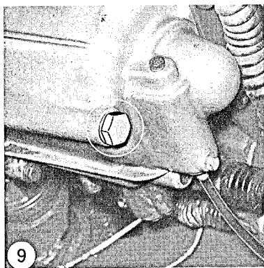
Bild 123 Getriebeölablaßschraube
