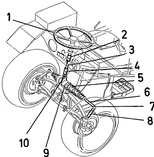
Bild 41 Lenkung
