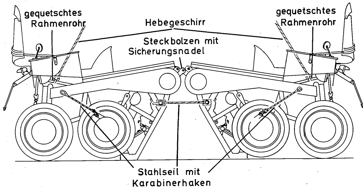
Bild 114 Verladen von zwei Fahrzeugen
