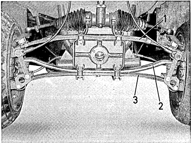
Bild 46 Federn
