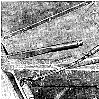
Bild 34 Handbremshebel
