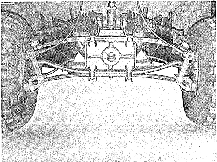
Bild 31 Vorderachse
