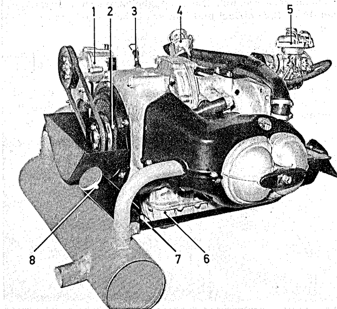
Bild 10 Motor rechts (bei ausgebautem Motor)
