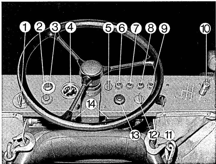
Bild 24 Instrumententafel
