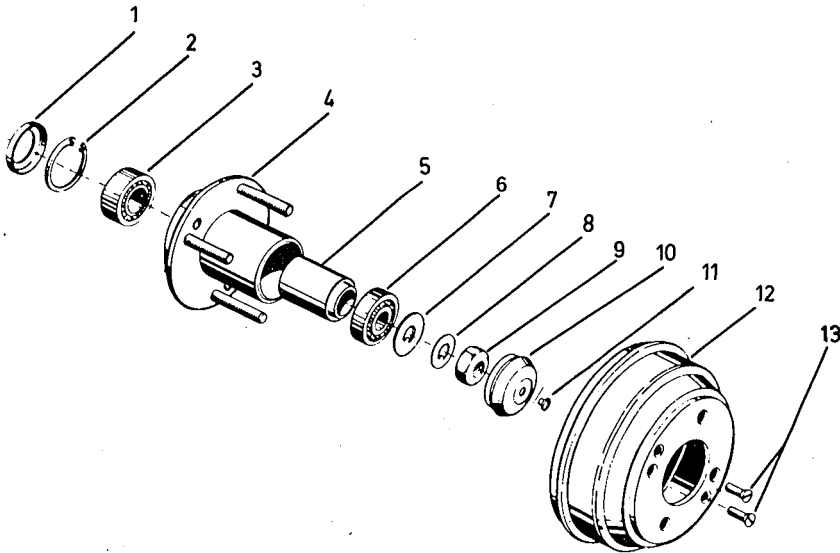
Bild 39 Vorderradnabe
