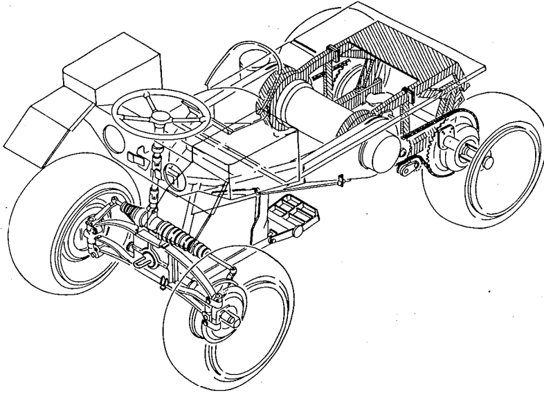
Bild 43 Fahrgestell, Hinterwagen
