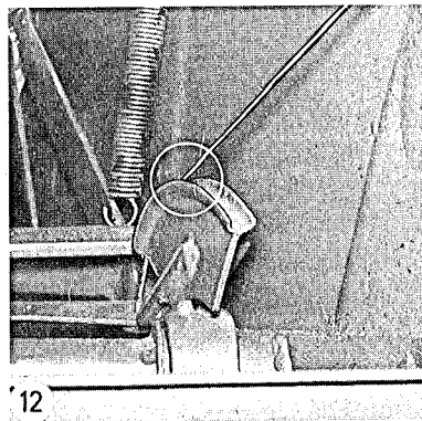
Bild 126 Seilzug für Gasbetätigung (am Gaspedal)
