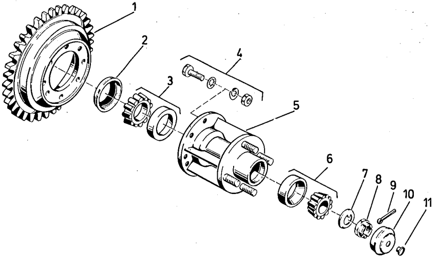
Bild 40 Hinterradnabe
