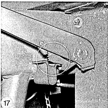
Bild 132 Handbremshebel
