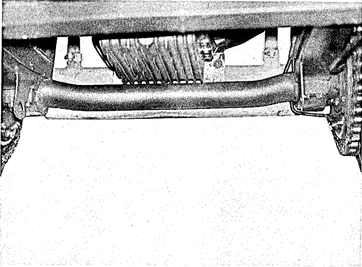
Bild 32 Hinterachse
