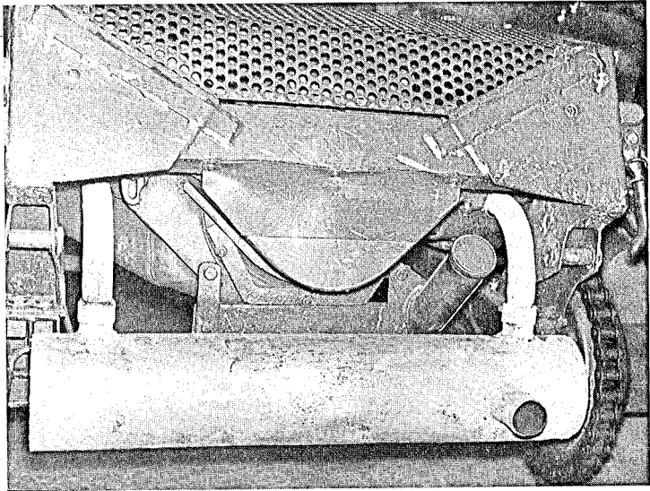
Bild 18 Auspuffanlage
