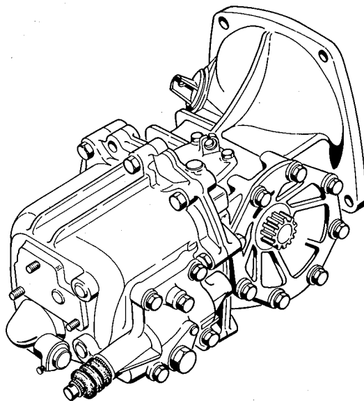
Bild 29 Wechsel- und Ausgleichgetriebe
